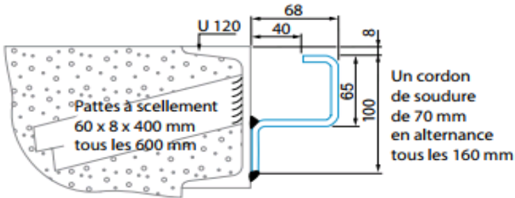
FIXATION DU RAIL KBS A SOUDER
